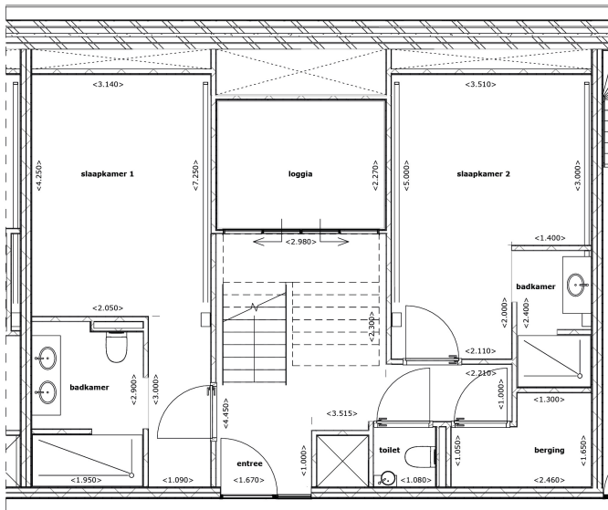
Plattegrond verdieping 03 1:50
