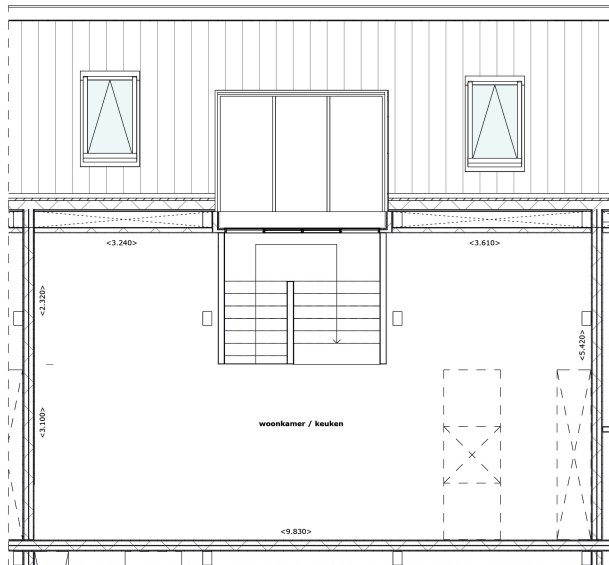
Plattegrond verdieping 04 1:50
